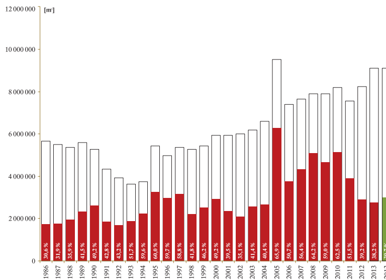
Obrázok 3. Podiel náhodných ťažieb (červená) na celkovom objeme ročných ťažieb s prognózou pre rok 2014 (odhad po spracovaní 55 % údajov)
