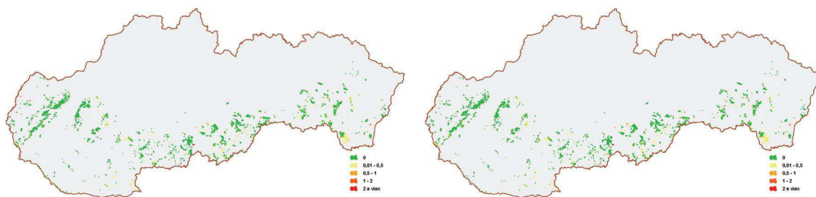
Obrázok 8. Početnosť znášok mnišky veľkohlavej v porastoch Slovenska v roku 2012 a 2013
