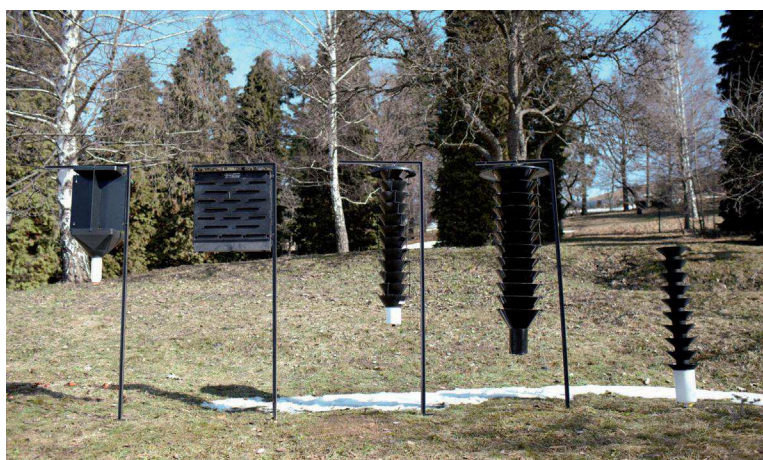
Obrázok 10. Rôzne konštrukčné typy feromónových lapačov na podkôrny hmyz: (zlava) Ekotrap, Teysohn, Lindgren funnel trap, Experimentálny prototyp, BEKA trap
